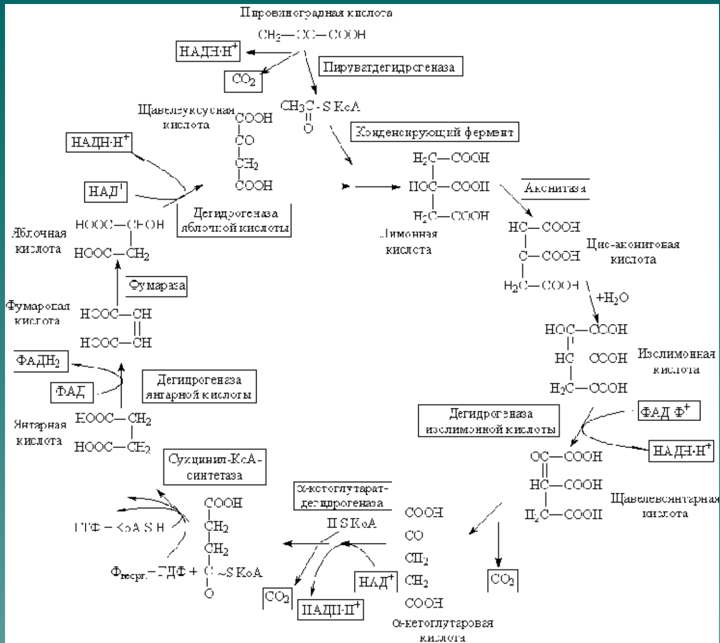
ЦИКЛ ТРИКАРБОНОВЫХ КИСЛОТ
