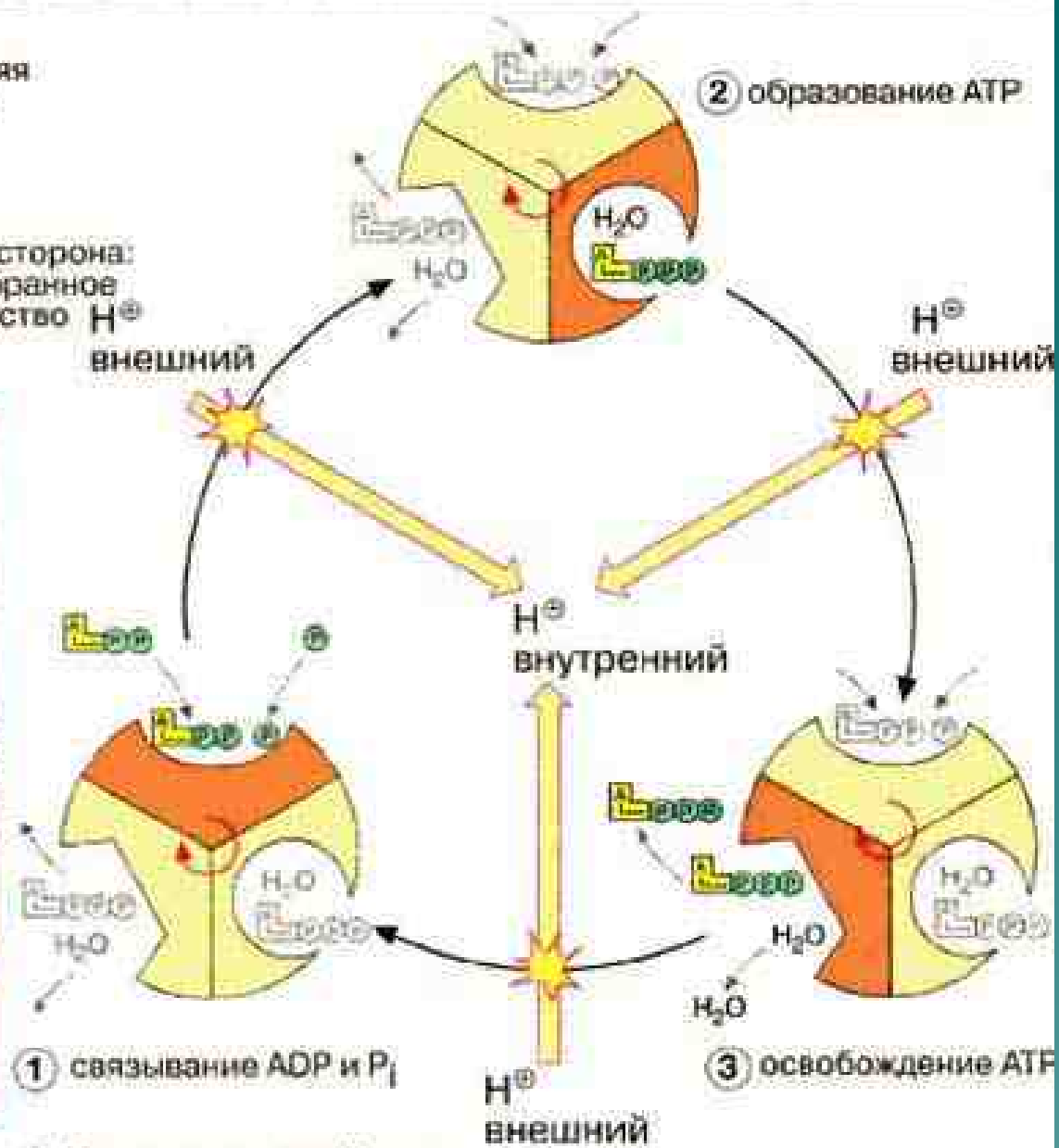
2. Каталитический цикл
