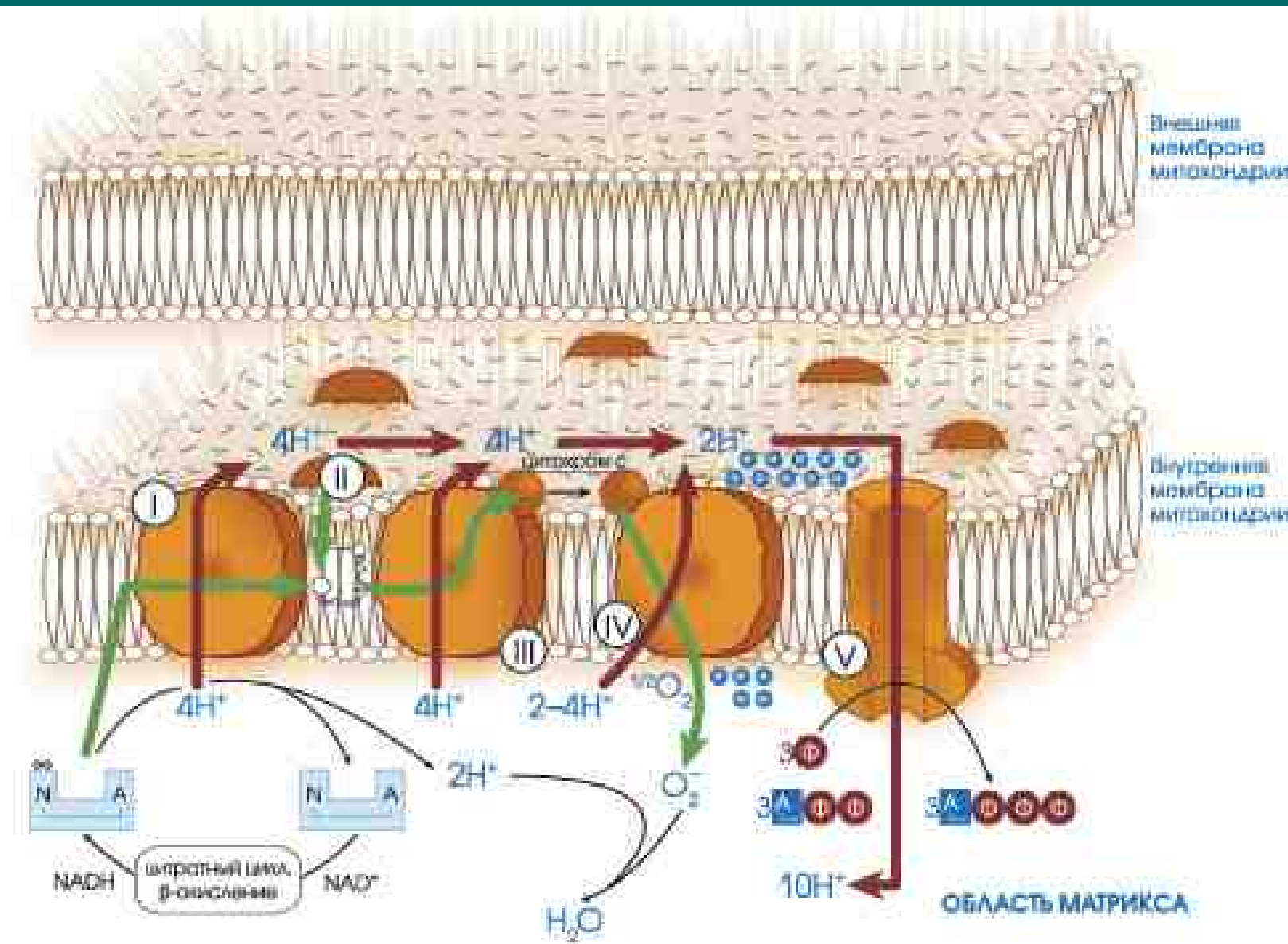
I – NADH-дегидрогеназа (убихинон); II – сукцинатдегидрогеназа; III – убихинол-цитохром c-редуктаза; IV – цитохром c-оксидаза; V – H^+ -транспортирующая АТФ-синтаза. — Поток электронов — Поток протонов
